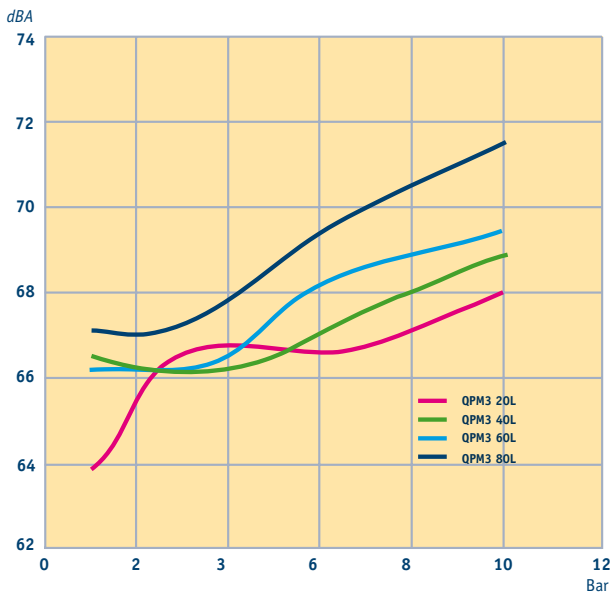
Geräuschemission QPM3-Pumpe
